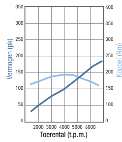
2.0i CVVT-motor Levert bij 6.200 t.p.m. een maximumvermogen van 120 kW/163 pk.
