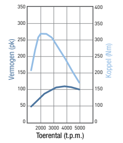
1.7 CRDi-motor Levert bij 4.000 t.p.m. een maximumvermogen van 85 kW/116 pk.
