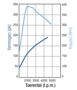
2.0 CRDi-dieselmotor Levert bij 4.000 t.p.m. een maximumvermogen van 135 kW/184 pk.
