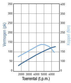
1.6 GDI-motor Levert bij 6.300 t.p.m. een maximumvermogen van 99 kW/135 pk.
