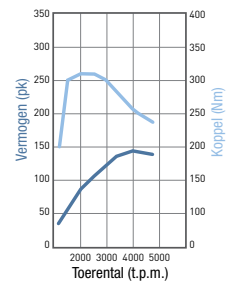
2.0 CRDi-dieselmotor Levert bij 4.000 t.p.m. een maximumvermogen van 100 kW/136 pk.
